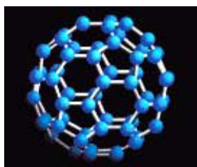
フラレンの代表格「C60」の分子構造イメージ
