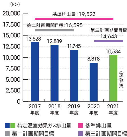
温室効果ガス排出量の推移
